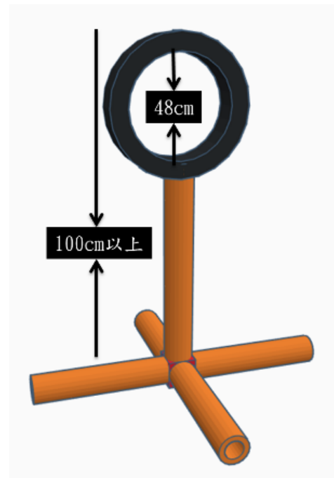
終點環
